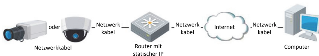
Abbildung 2–10 Zugriff auf die Kamera über einen Router mit statischer IP
