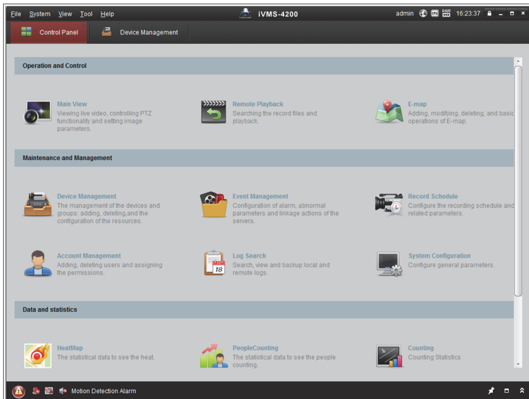
Abbildung 3–2 ivMS-4200 Systemsteuerung
